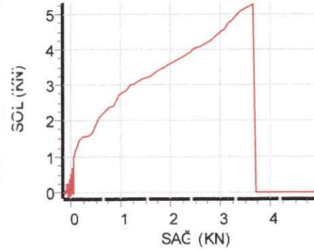
Ön Sol - Sağ Fren Dengesi
