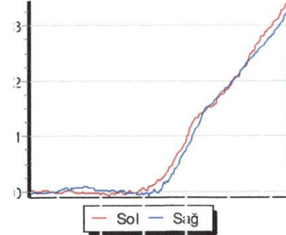
Arka Fren Kuvvetleri
